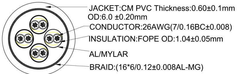
SEC:A-A
