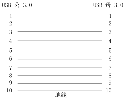
USB 公 3.0 转 USB 母 3.0 连线方式
